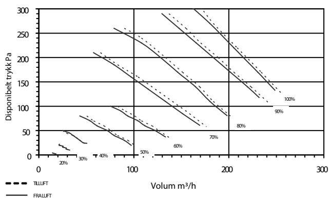
Spesifikke kurver for Piccolo eco med EU7/EU5 filter
